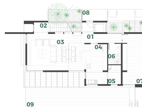
Planta baja
